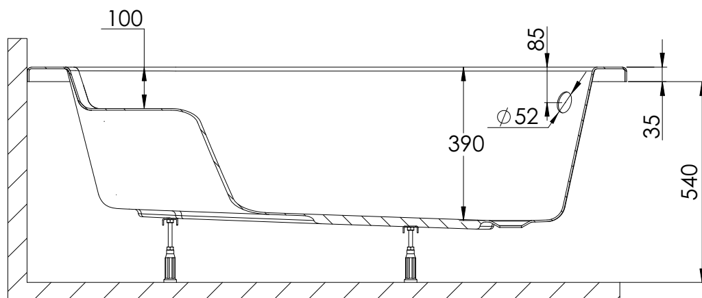
ŘEZ A-A
