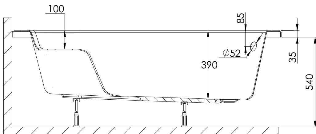
ŘEZ A-A
